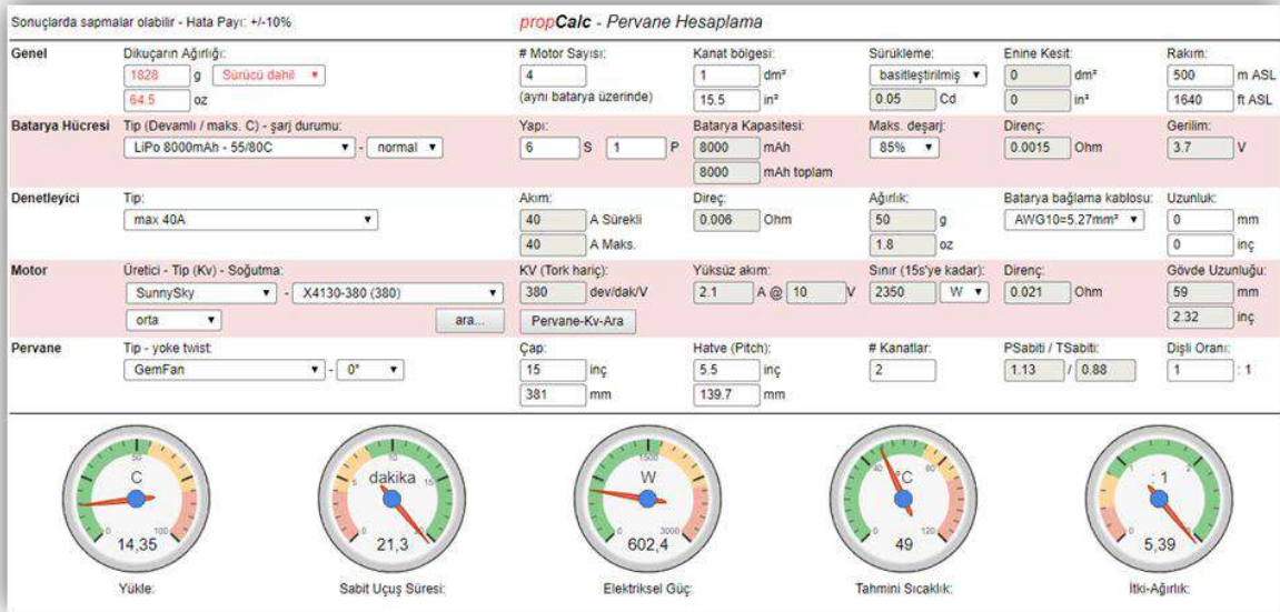
Şekil 6: Yeni tasarımla beraber uçuş süresi ( https://www.ecalc.ch/motorcalc.php ).
