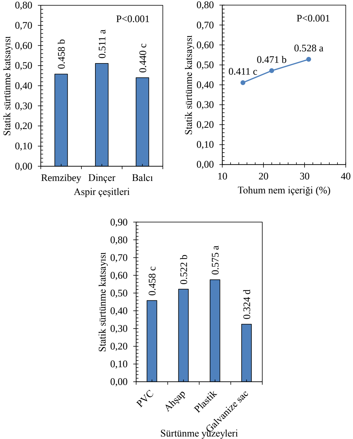
Şekil 3.1. Statik sürtünme katsayısının çeşit, nem ve sürtünme yüzeylerine göre değişimleri
