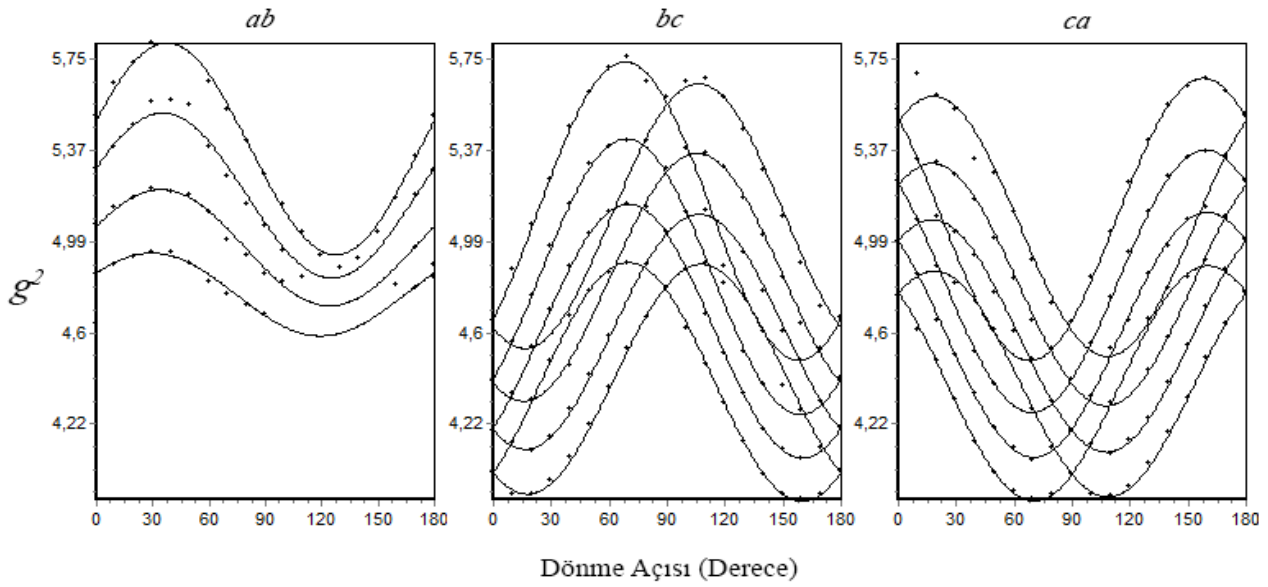
Şekil 2. \text{Cu}^{2+} katkılandırılmış [\text{Ni}(\text{sac})_2(\text{enc})_2].(\text{H}_2\text{O})_2 kristalinin oda sıcaklığındaki EPR spektrumlarının açısal değişimi.
