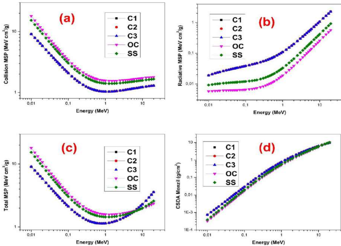
Şekil 1. 0.01-20 MeV enerji aralığında elektronlar için etkileşme parametreleri (a) Çarpışma MSP, (b) Işımalı MSP, (c) Toplam MSP (d) Menzıl
