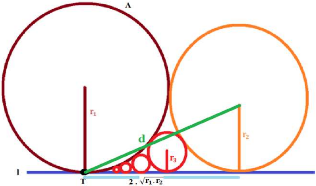
Şekil 7: Her çemberin l doğrusuna teğet noktaları arasındaki uzunluğu Pisagor bağıntısıyla bulduk.n.çemberle A çemberi arasındaki uzaklık 2\sqrt{r_1 \cdot r_n} dir.
