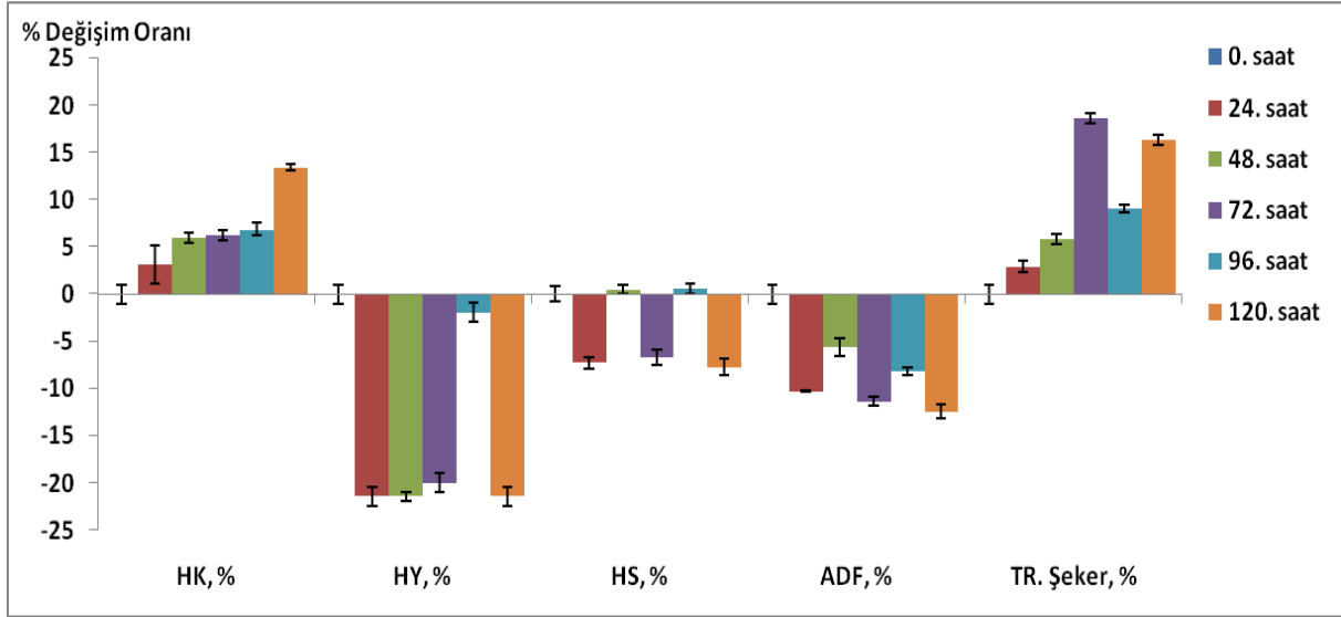
Şekil 2. ATK'nın fungal fermantasyonu sonucunda besin madde içeriğinde meydana gelen değişim
