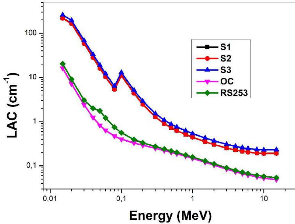
Şekil 2. Ni-katkılı bismut borat camlar (S1, S2 ve S3) ve karşılaştırma numuneleri (OC ve RS 253) için uyarıcı foton enerjisinin fonksiyonu olarak lineer azaltma katsayılarının değişim eğrisi.
