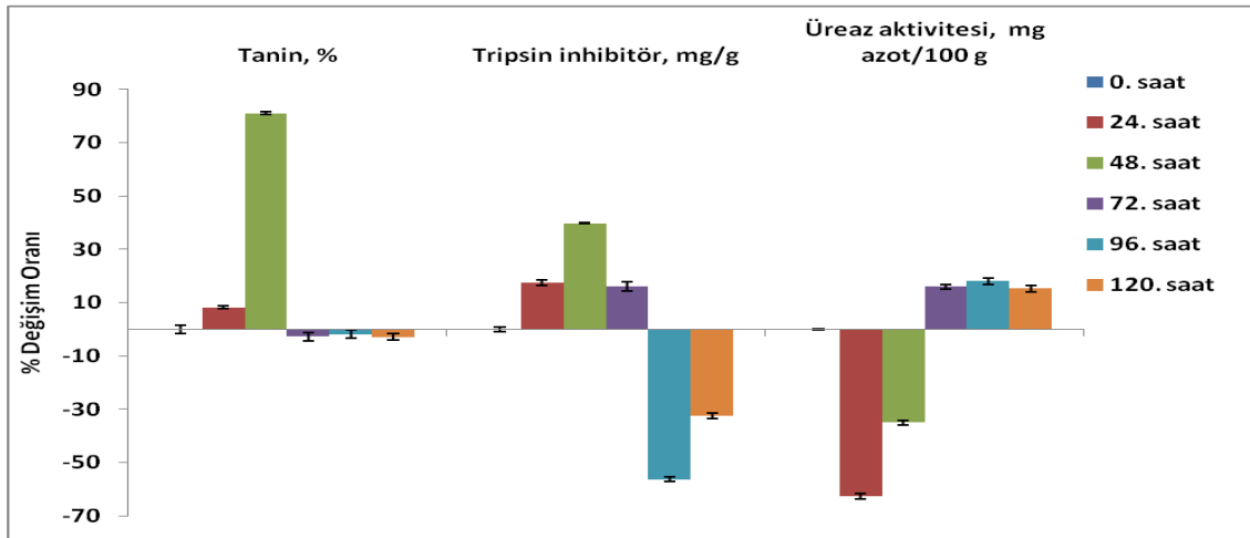
Şekil 3. SFK'nın fungal fermentasyonu sonucunda antibesinsel bileşiklerde meydana gelen değişim
