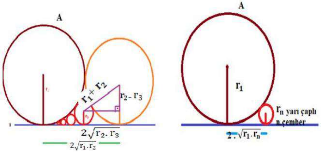
Şekil 7: Her çemberin l doğrusuna teğet noktaları arasındaki uzunluğu Pisagor bağıntısıyla bulduk.n.çemberle A çemberi arasındaki uzaklık 2\sqrt{r_1 \cdot r_n} dir.
