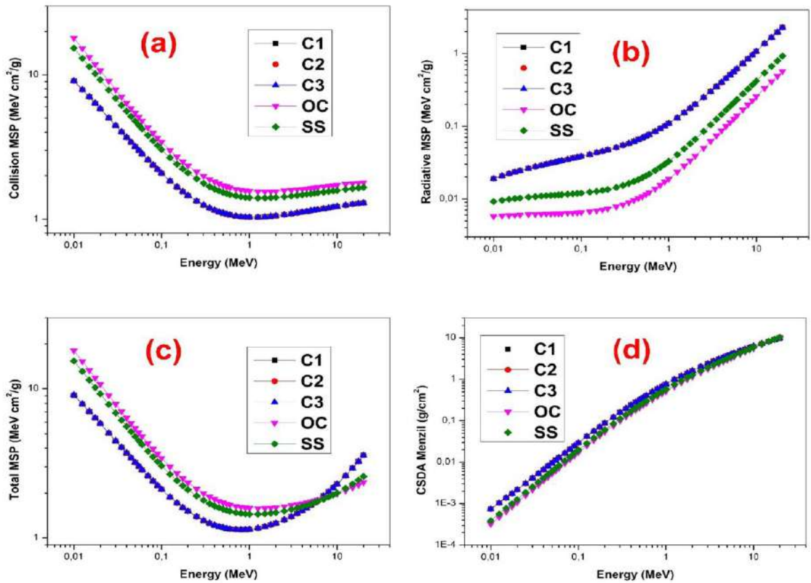
Şekil 1. 0.01-20 MeV enerji aralığında elektronlar için etkileşim parametreleri (a) Çarpışma MSP, (b) Işımalı MSP, (c) Toplam MSP (d) Menzil
