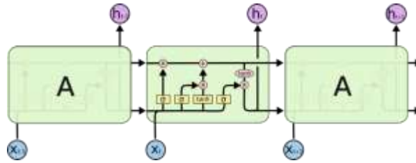
Şekil 1. LSTM yapısı ve katmanları
