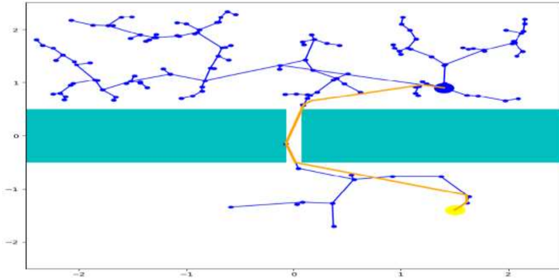
Fig. 6. RRT Path Extend
